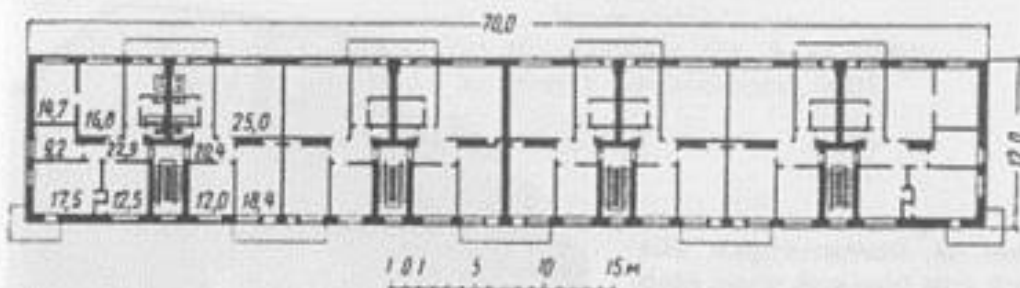
Рис. 31. Магнитогорск. План типового этажа жилого дома центральной зоны квартала № 1 соцгорода (тип Госпроекта). Источник: Казаринова В.И., Павличенков В.И. Магнитогорск. М., 1961. С. 151
